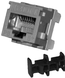
Модуль GigaFlex PS6+ категории 6, AX101067
