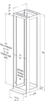
Серверная стойка BSR-8419
