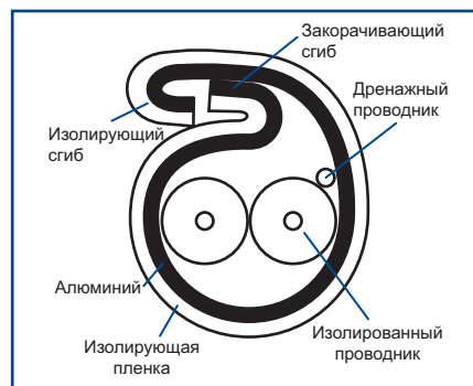
Рис. 3: Экран из фольги со сгибом типа Z снижает уровень наводок в многопарных кабелях.
