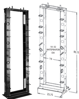
Кабельная стойка 84" (2.13 м) типа BCR-8419
