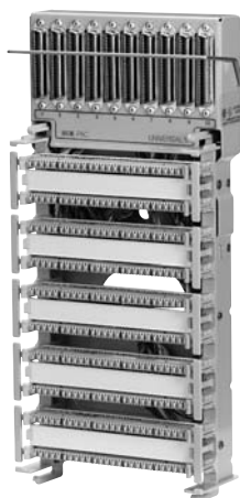
Универсальная система ВІХ-РАС, А0321776, 10-10
