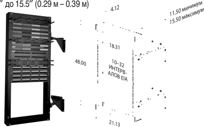
Кронштейн типа AX100785 для крепления к стене, 2U
