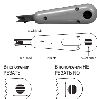
Инструмент для заделки кабеля BIX A0270165
