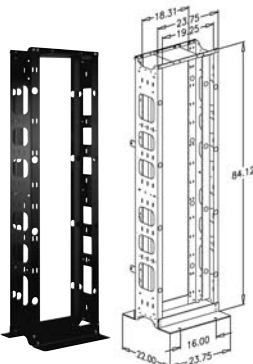
Кабельная стойка типа BCR-8419-10: 84" (2.13 м) с 10" каналом
