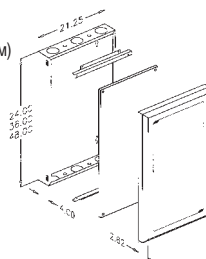
BWM-9312-1600 Блок вентиляторов: (2) вентилятора диаметром 4" (0.10 м) (160 куб. фут./мин.) с защитной решеткой
