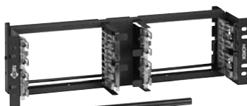
Монтажный набор GigaBIX, 48 портов, AX101985
